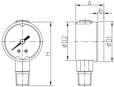
Φ40~Φ98径向
