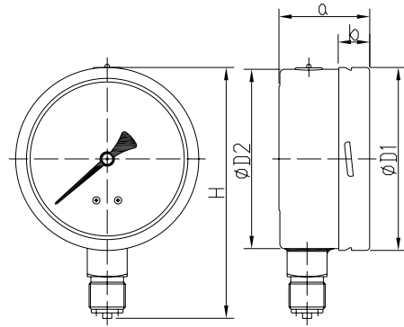
Φ63~Φ250内卡式径向
