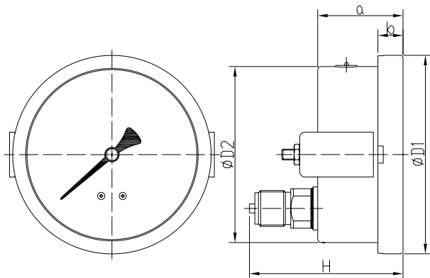
Φ100外卡式下轴向带卡子
