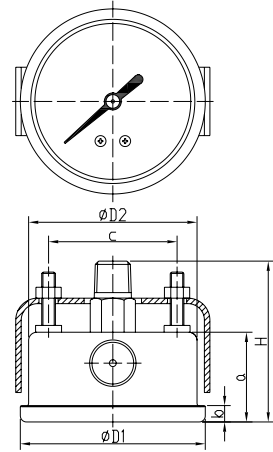
Φ63、Φ98中轴向卡子
