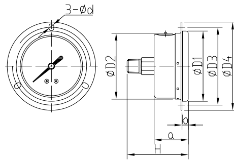
Φ63、Φ98中轴向前边
