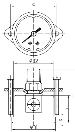
Φ43、Φ53中轴向卡子
